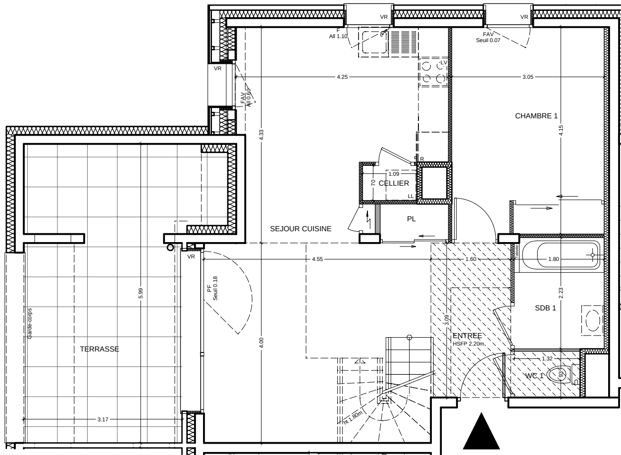
NIVEAU R+2
