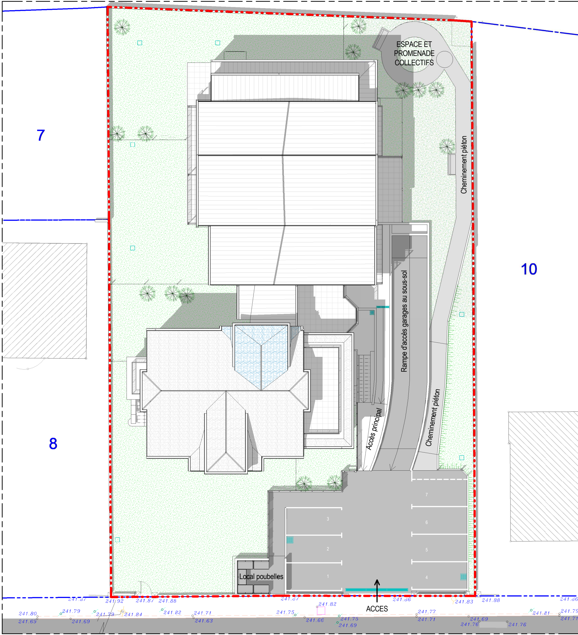
1 Plan de Masse vente Ech : 1 : 200
